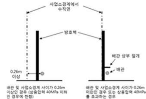
[ 그림 3 ] 고압가스설비 상부 차폐방법
