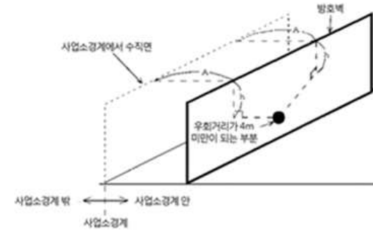
[ 그림 2 ] 방호벽의 높이 측정방법
