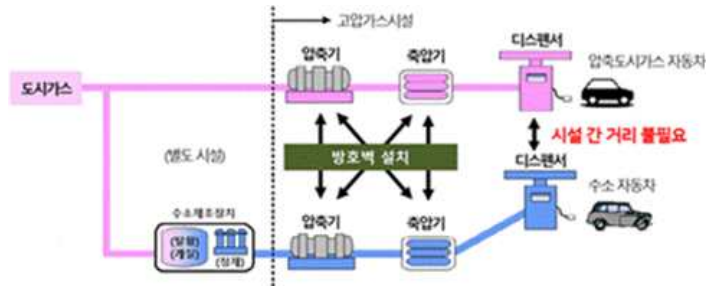
[ 그림 1 ] 고압가스설비 간 이격거리 개념
