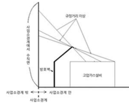
[ 그림 1 ] 차폐방법
