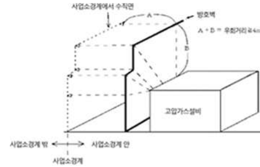
[ 그림 1 ] 우회거리 측정방법
